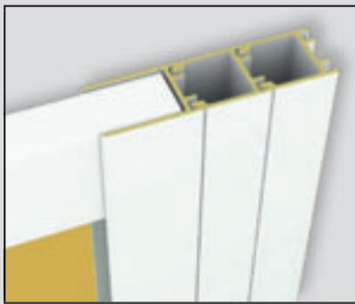
Použití 2 ks prodlužovacích profilů Vám poskytne rozšíření výsledného rozměru zástěny až o 45 mm. Při použití dvou částí prodlužovacích profilů zůstává pevnost sprchové (nebo vanové) zástěny stejná.
