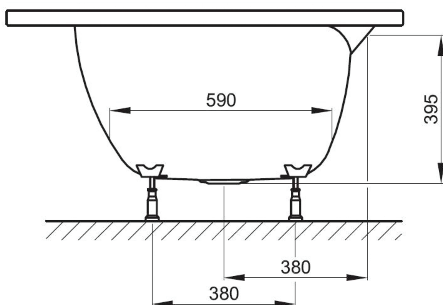
Výkres: Roh vlevo, obj. č. 6056
